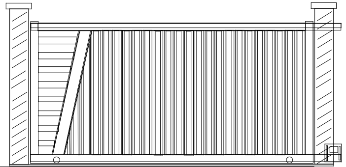
6- Plein Vertical avec Ajouré Latéral montant incliné Tarif A de base + 1 montant oblique
