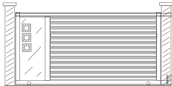
7- Plein Horizontal avec panneau lisse + déco. Latéral Tarif A de base + 1 montant droit + 3 décorations carrées
