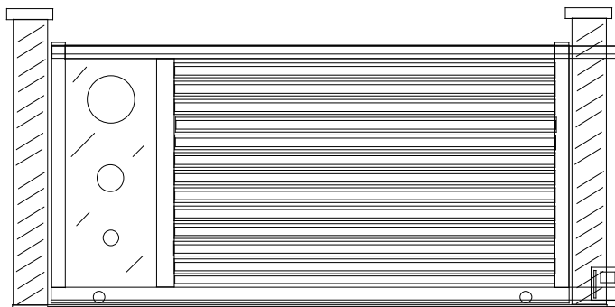
5- Plein Horizontal avec panneau lisse + déco. Latéral Tarif A de base + 1 montant droit + 3 décorations rondes
